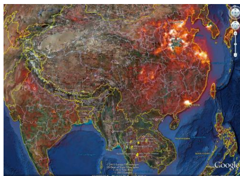
Luchtvervuiling Azië 2006
